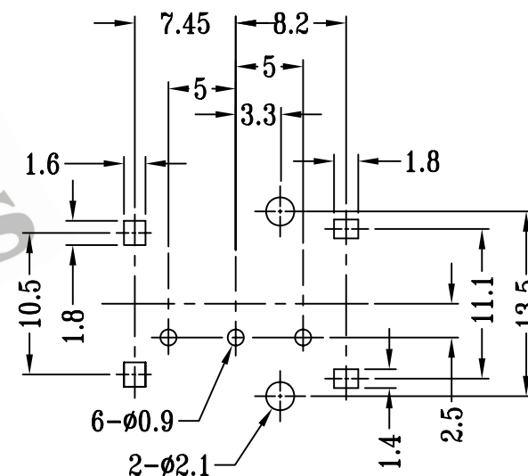
P.C.B LAYOUT
